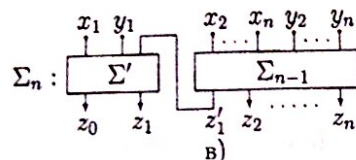
Рис. 22. Схема сумматора \Sigma_n
